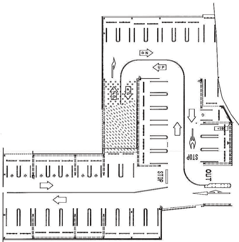
1階平面图
