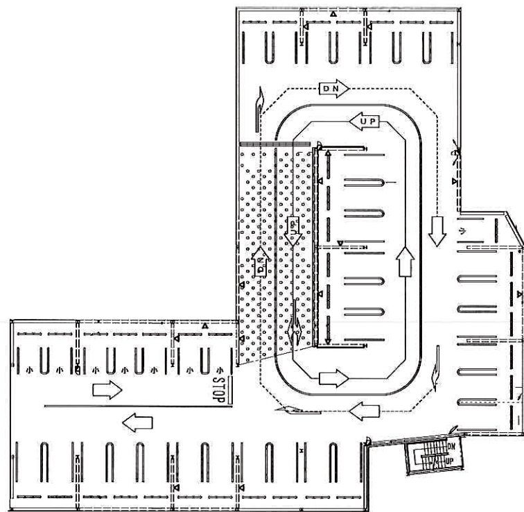
2階平面图
