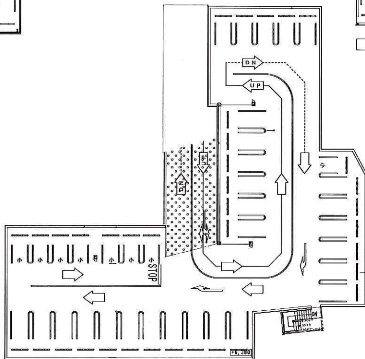
R階平面图
